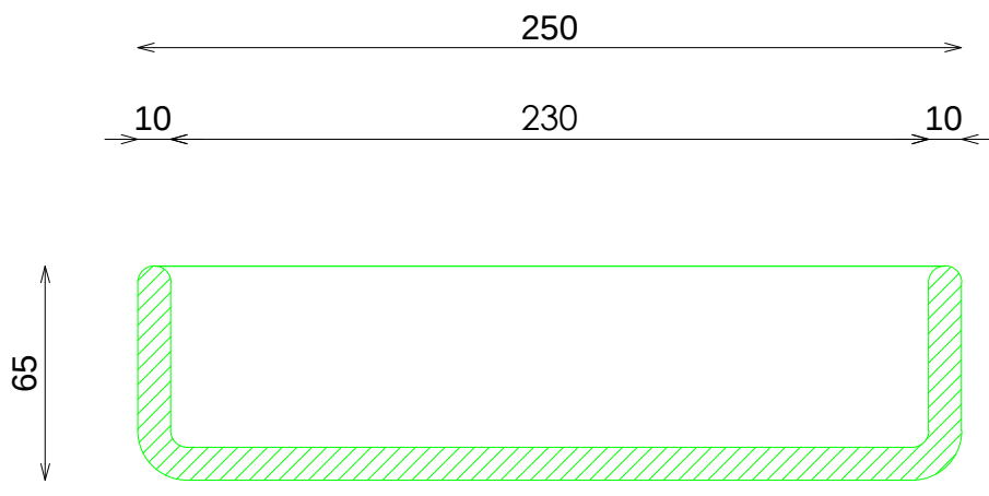
PERFIL
