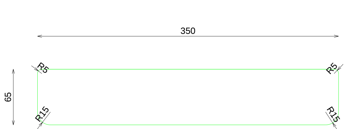
ALZADO
