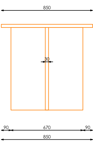
ALZADO IZQUIERDA
