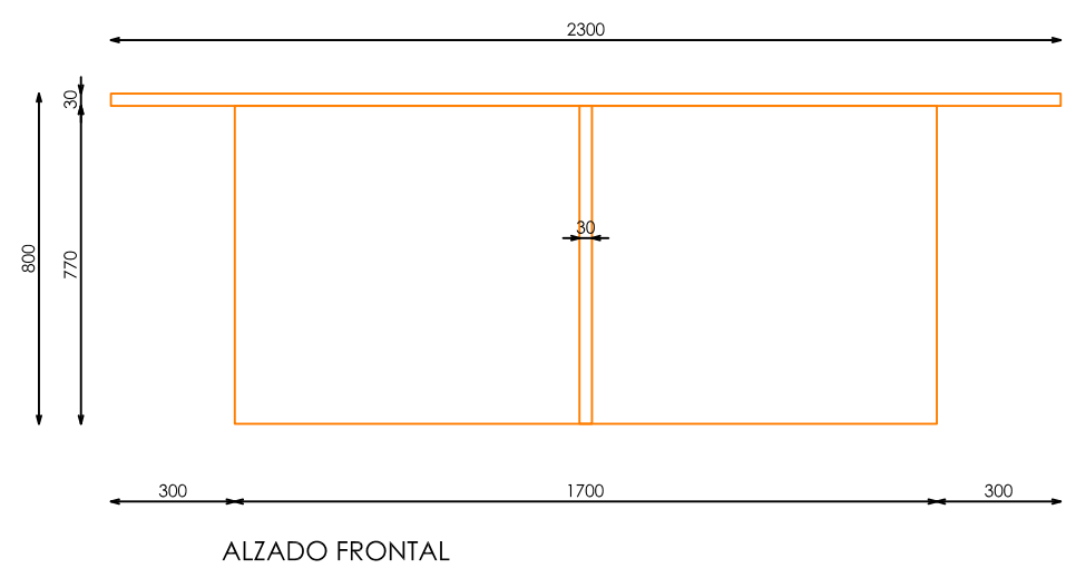
ALZADO FRONTAL
