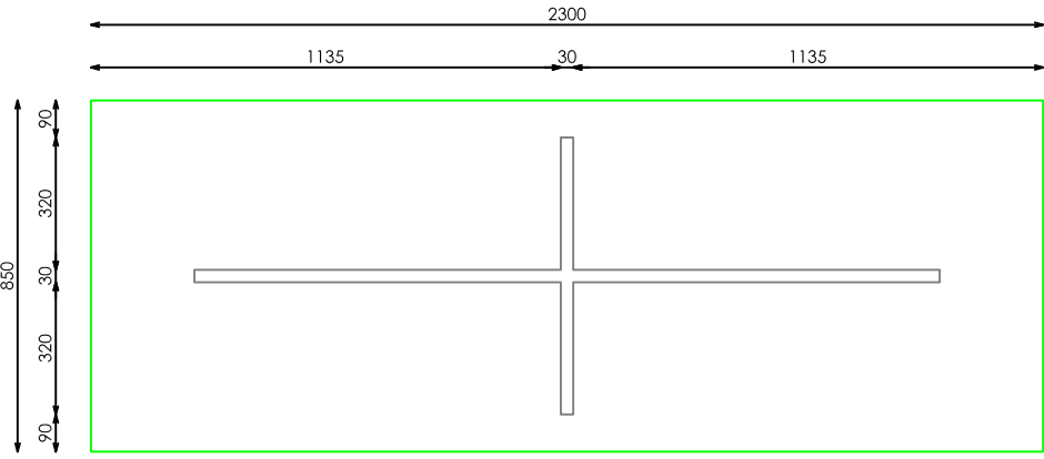
PLANTA
