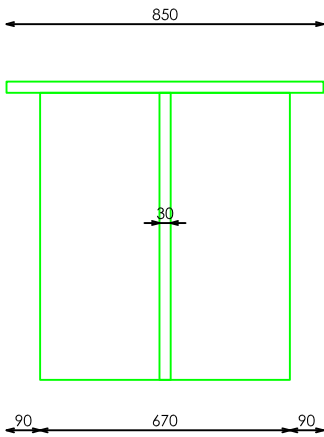
ALZADO IZQUIERDA
