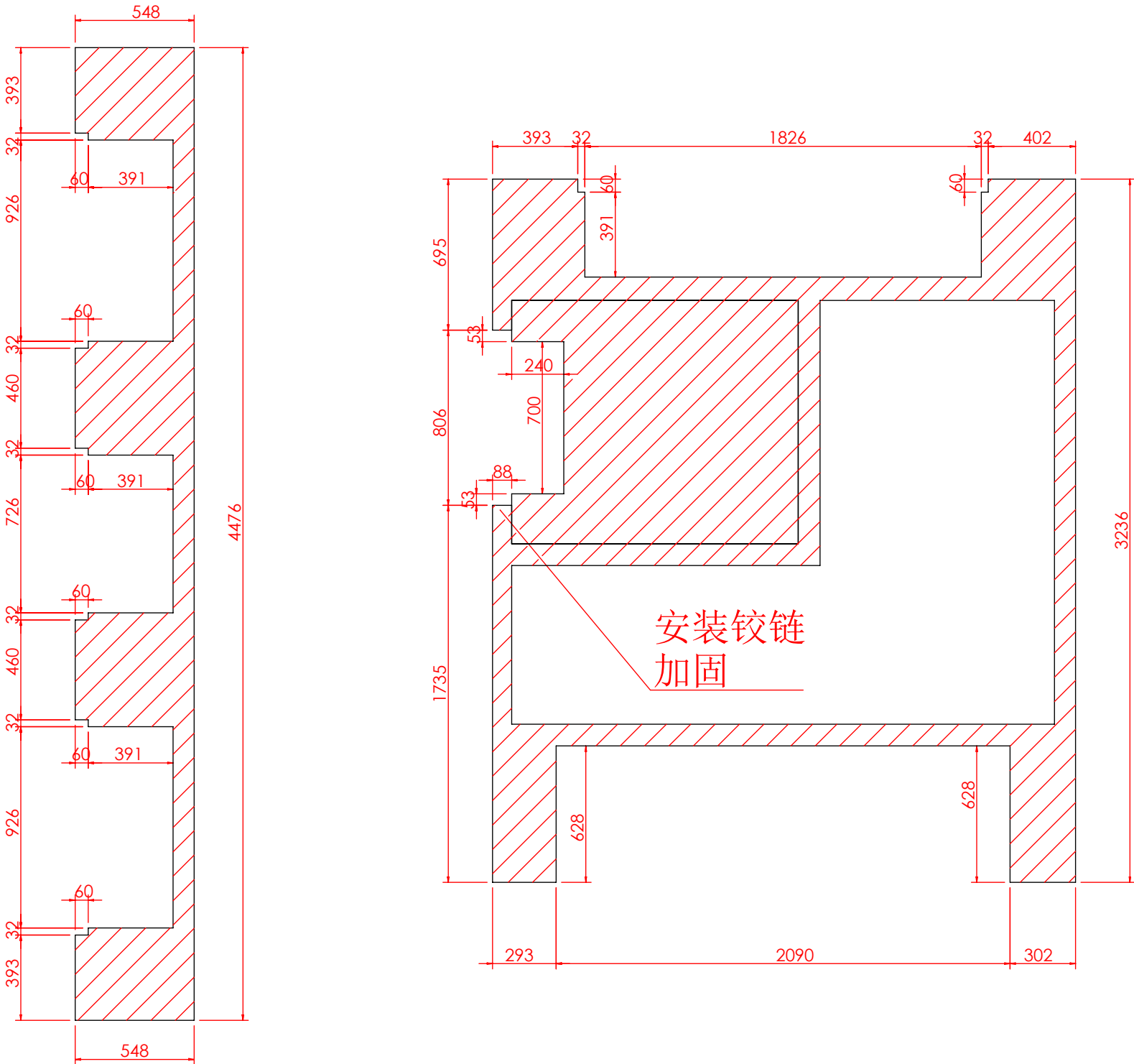
剖面 AJ-AJ
