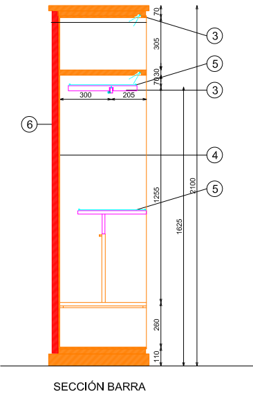
SECCIÓN BARRA
