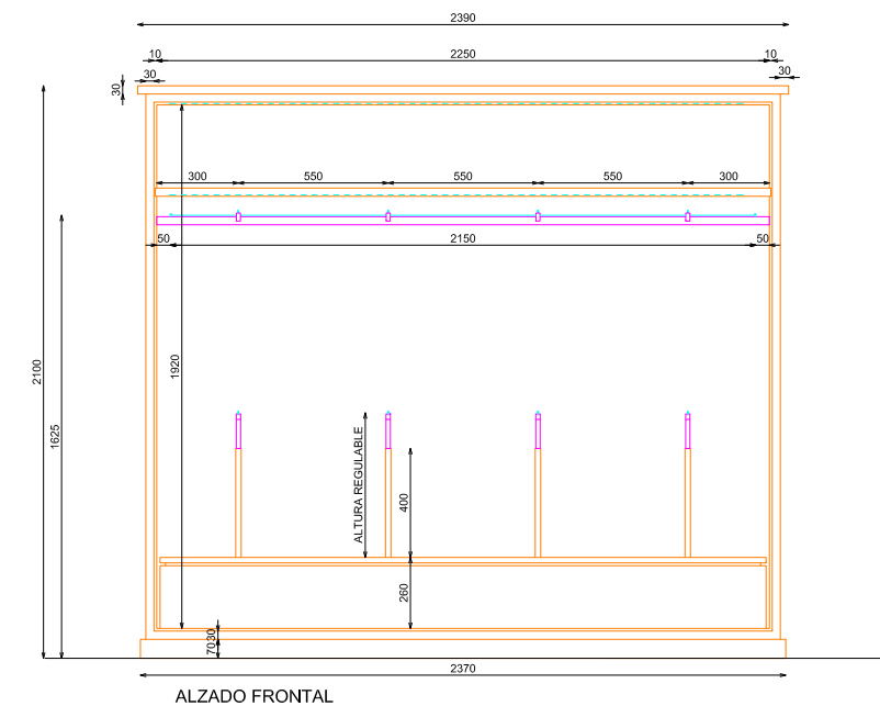
ALZADO FRONTAL
