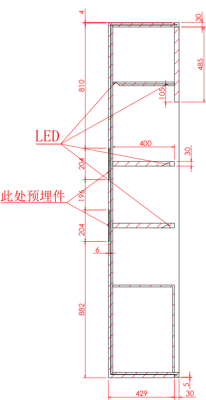
剖面 AH-AH
