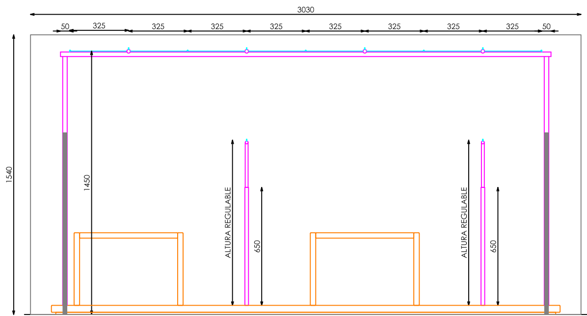
ALZADO FRONTAL
