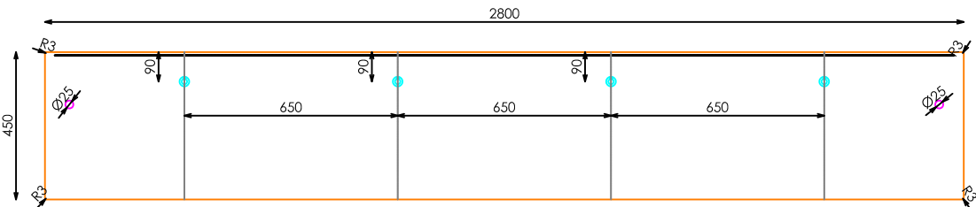
PLANTA TARIMA
