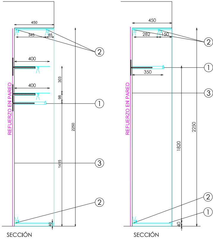
SECCIÓN
