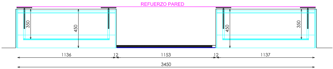
PLANTA
