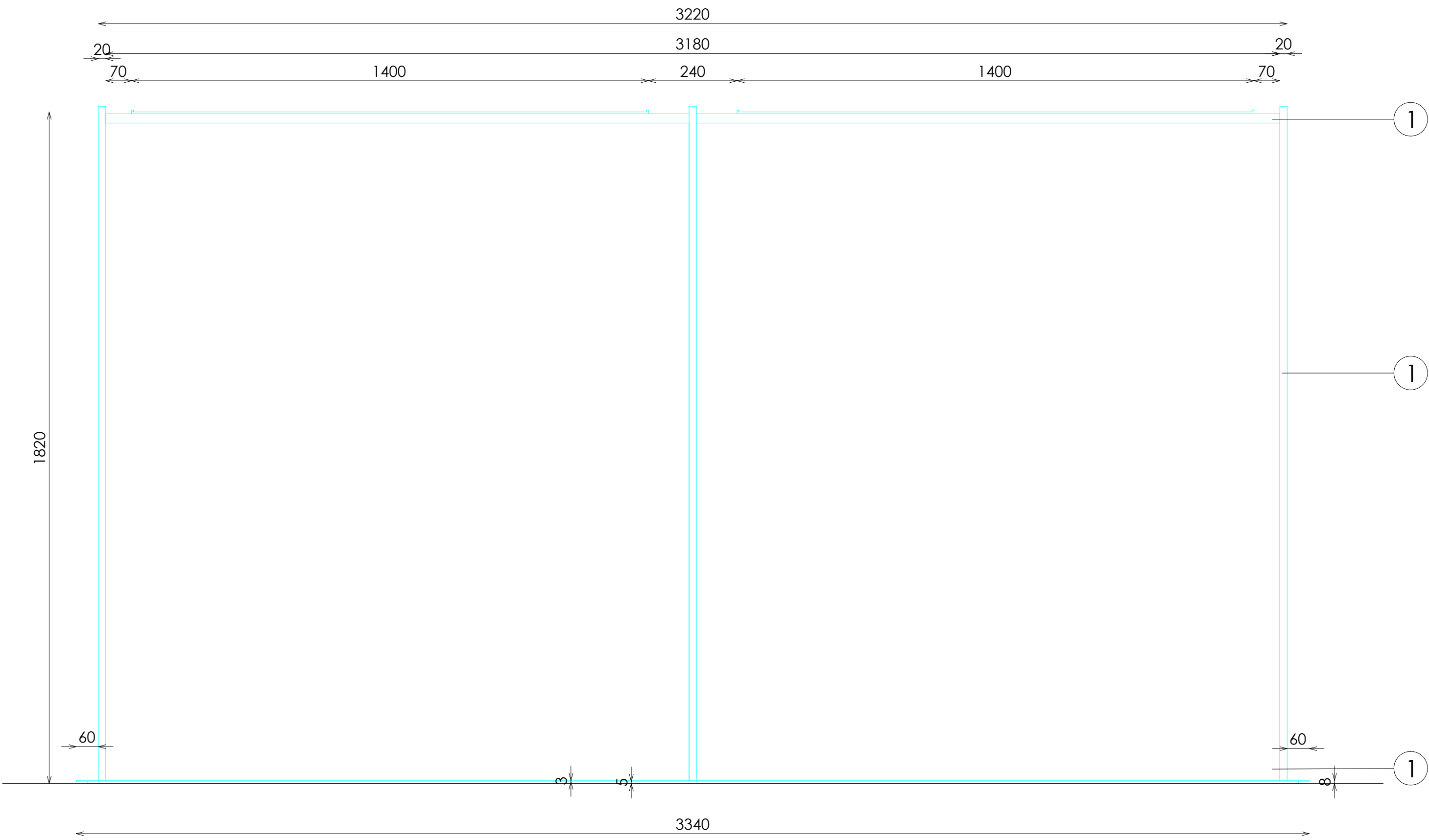
ALZADO SECCIONADO
