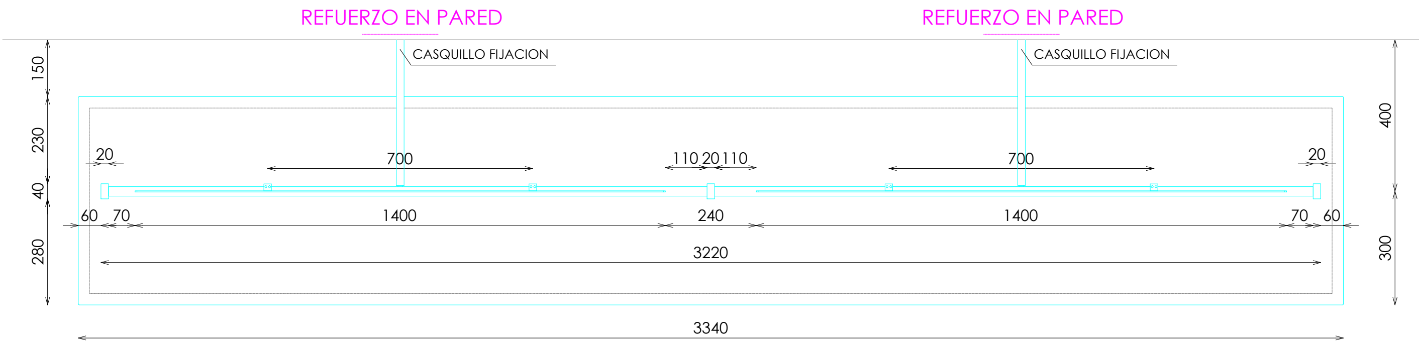
PLANTA
