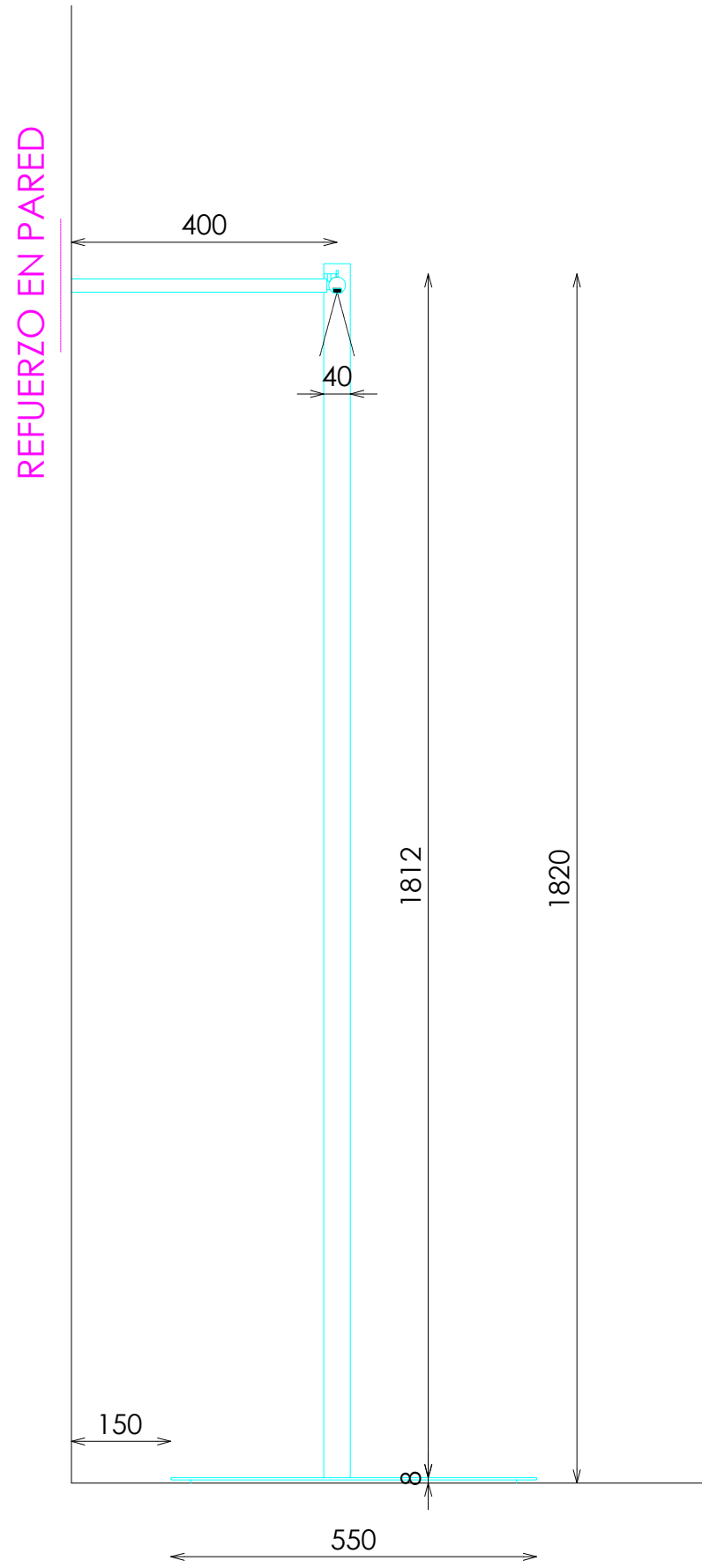
PERFIL SECCIONADO
