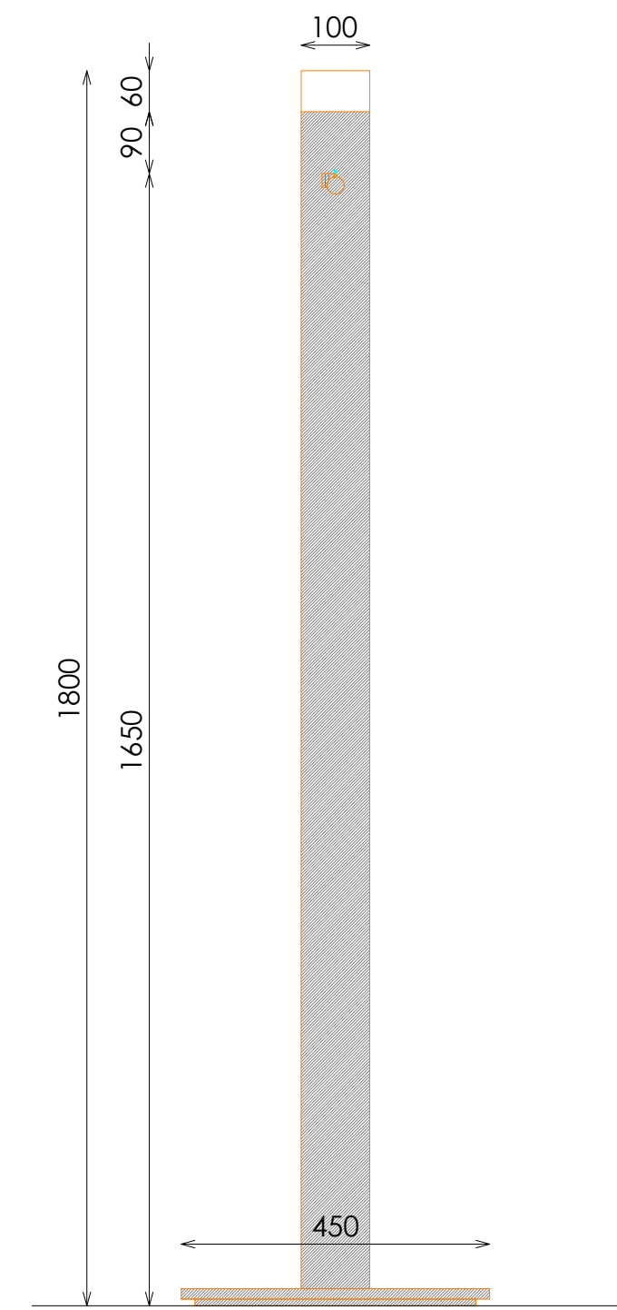
SECCION
