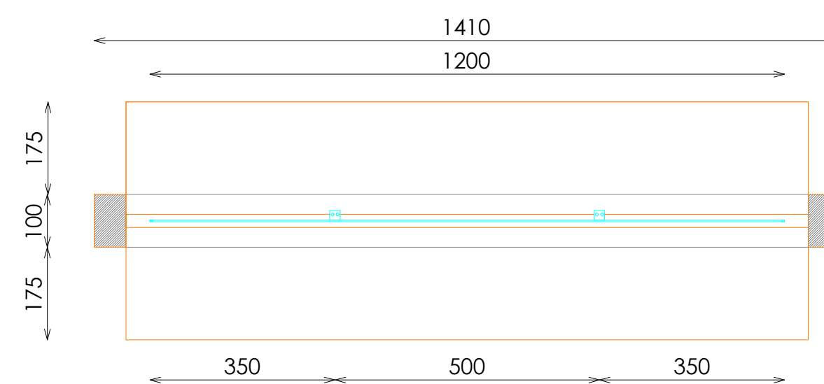
PLANTA SECCIONADA
