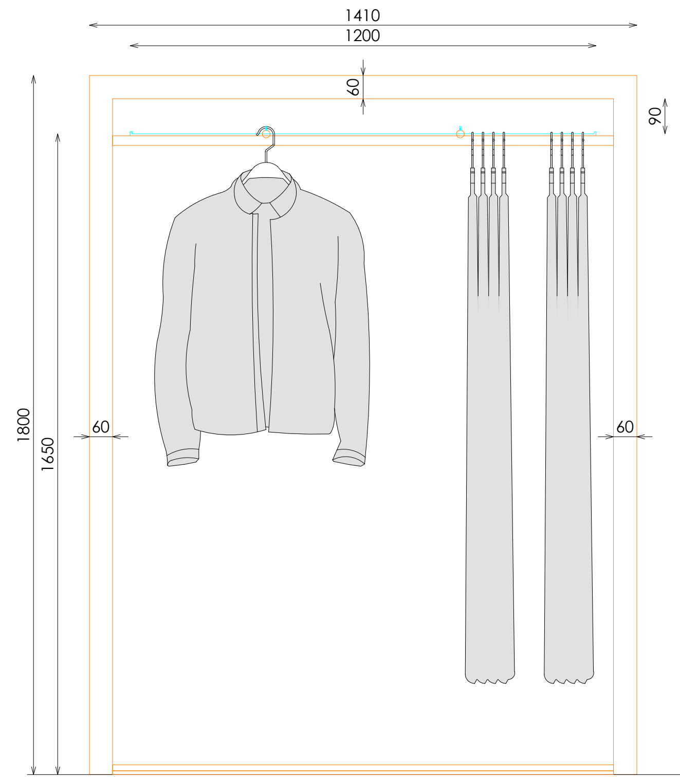
ALZADO
