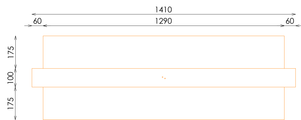
PLANTA
