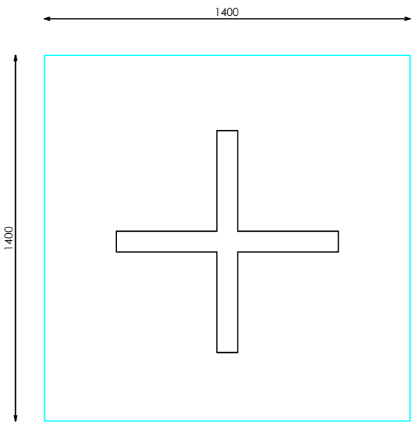
PLANTA
