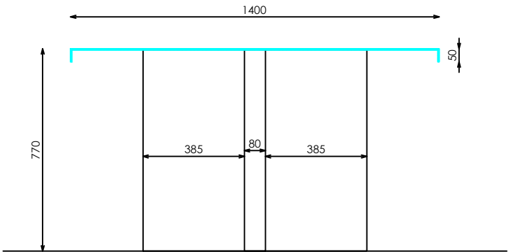
ALZADO LATERAL
