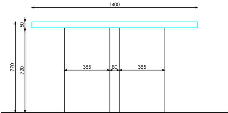
ALZADO FRONTAL
