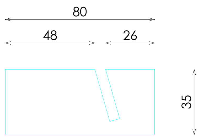
SECCIÓN
