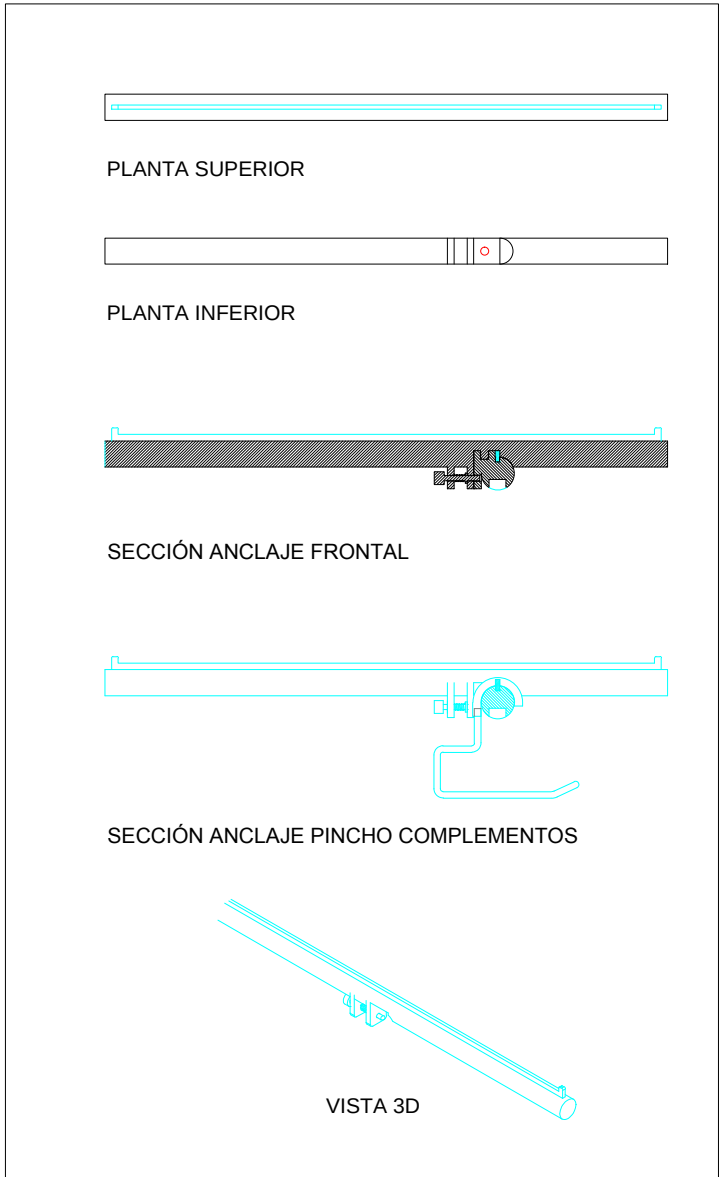
DETALLE ANCLAJE PINCHO COMP.
