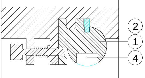
DETALLE ANCLAJE FRONTALES EXTRAIBLES
