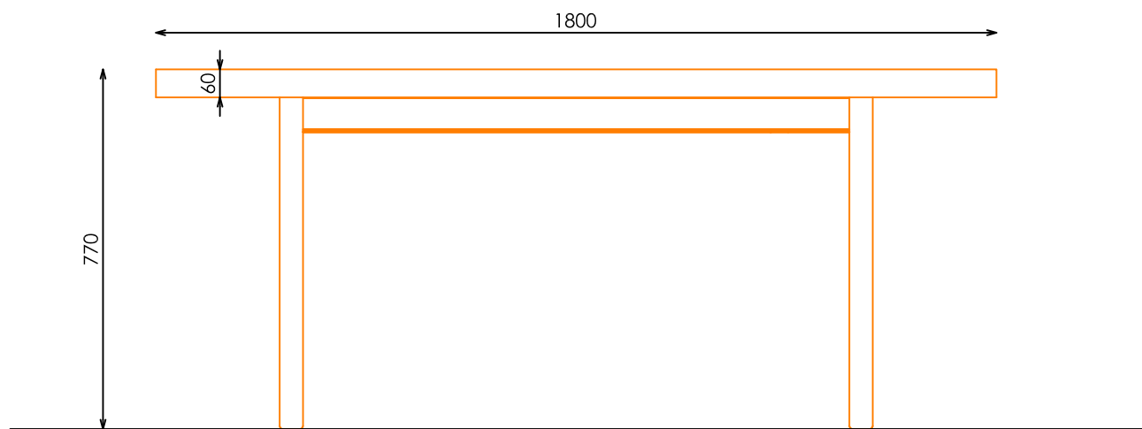
ALZADO
