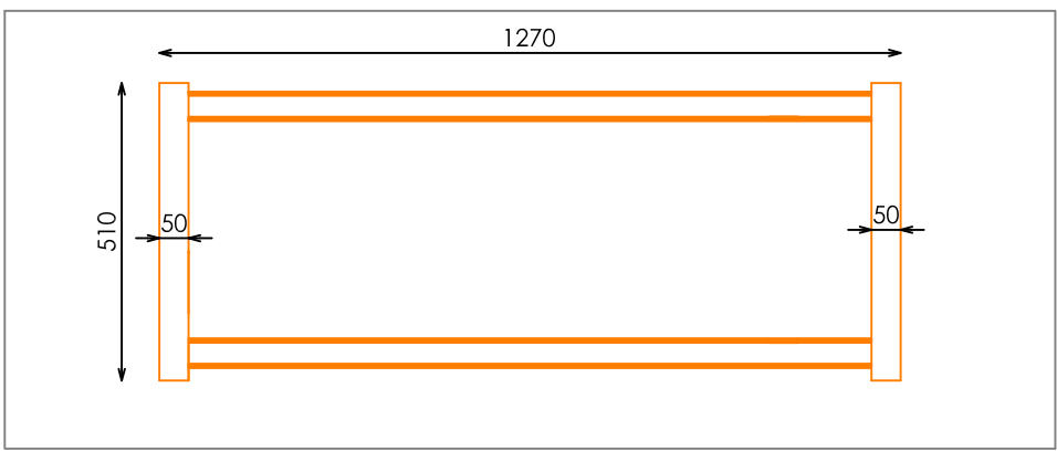
PLANTA (PATAS)
