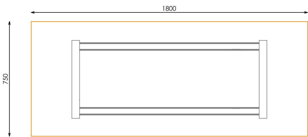
PLANTA
