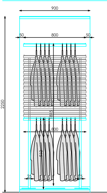
ALZADO
