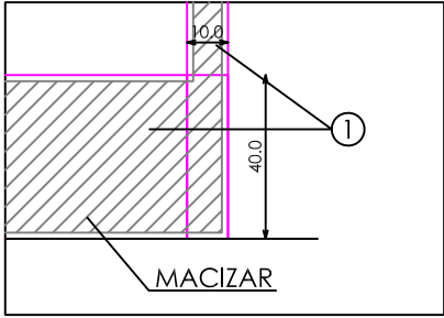
DETALLE C
