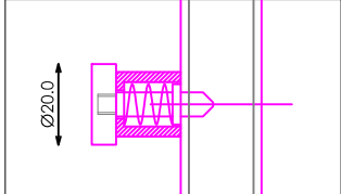
DETALLE SISTEMA ANCLAJE
