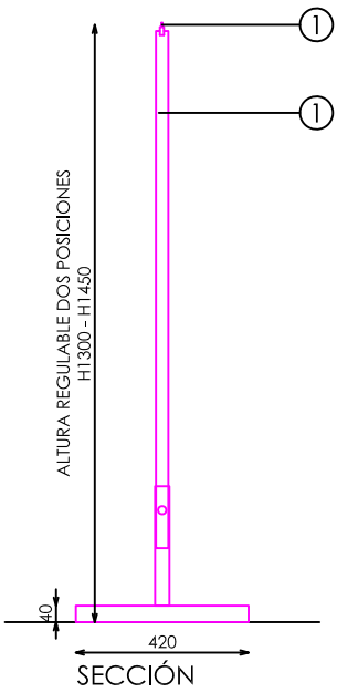
SECCIÓN
