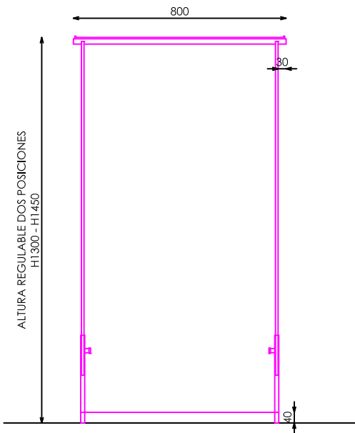
ALZADO
