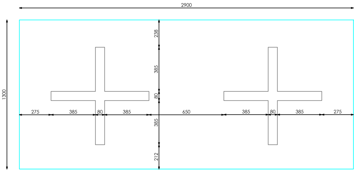
PLANTA
