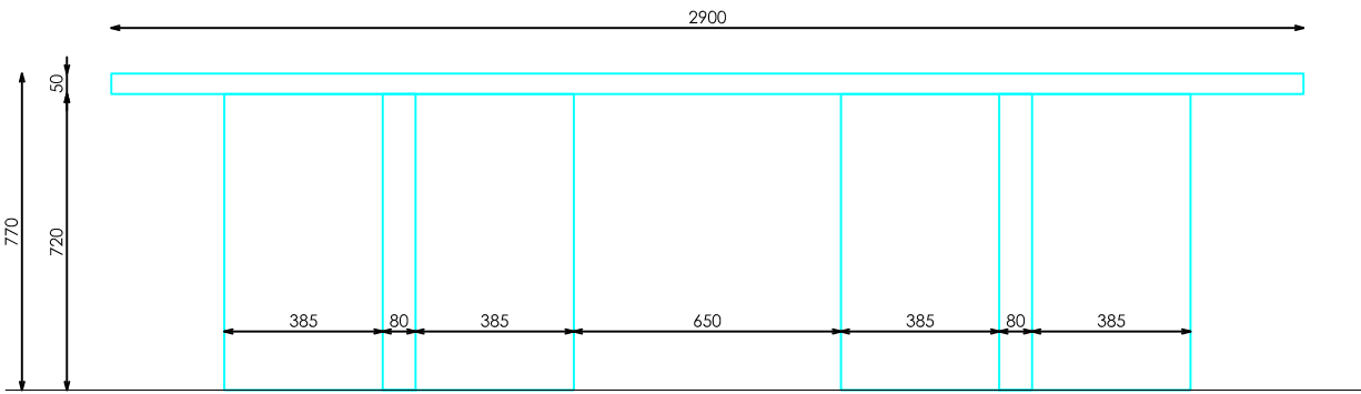
ALZADO FRONTAL
