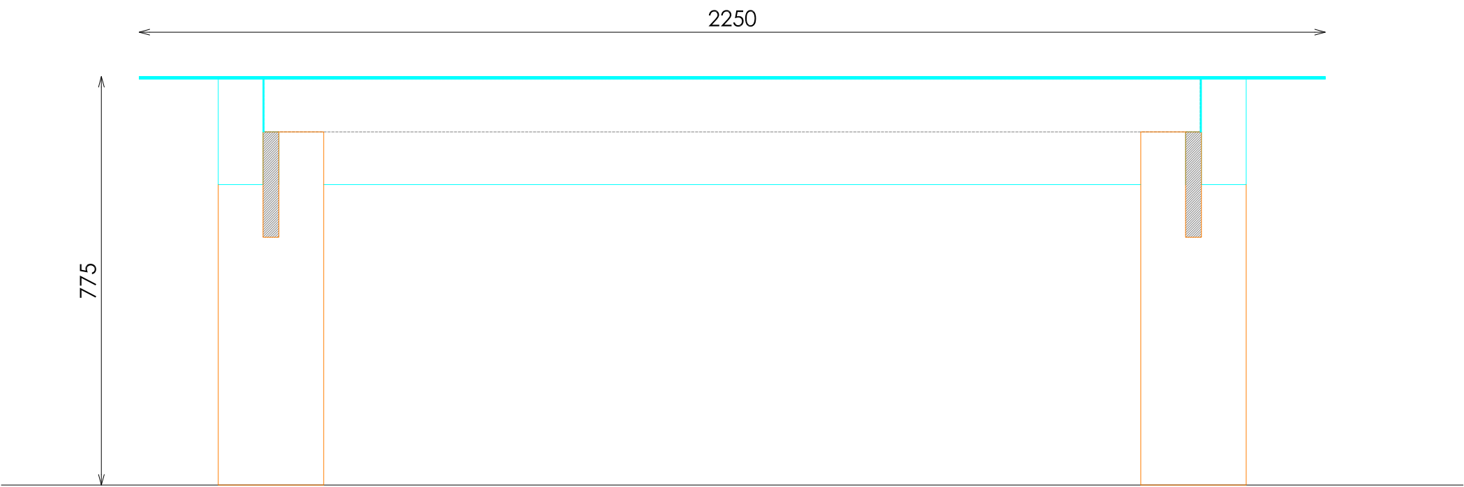
SECCIÓN LONGITUDINAL
