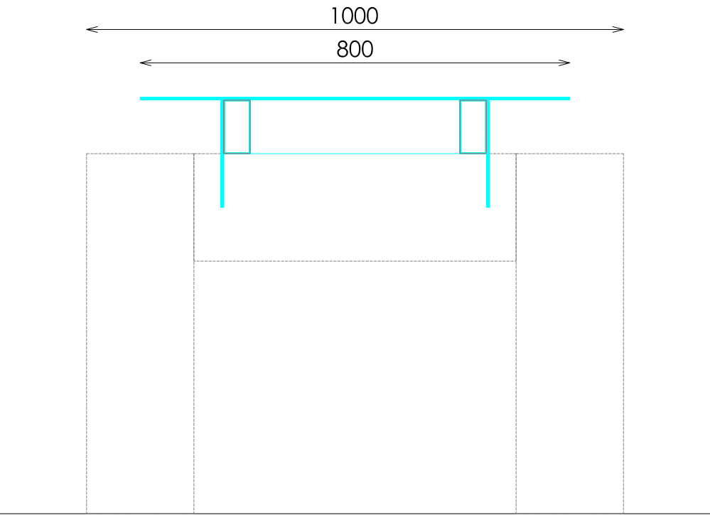
SECCIÓN TRANSVERSAL
