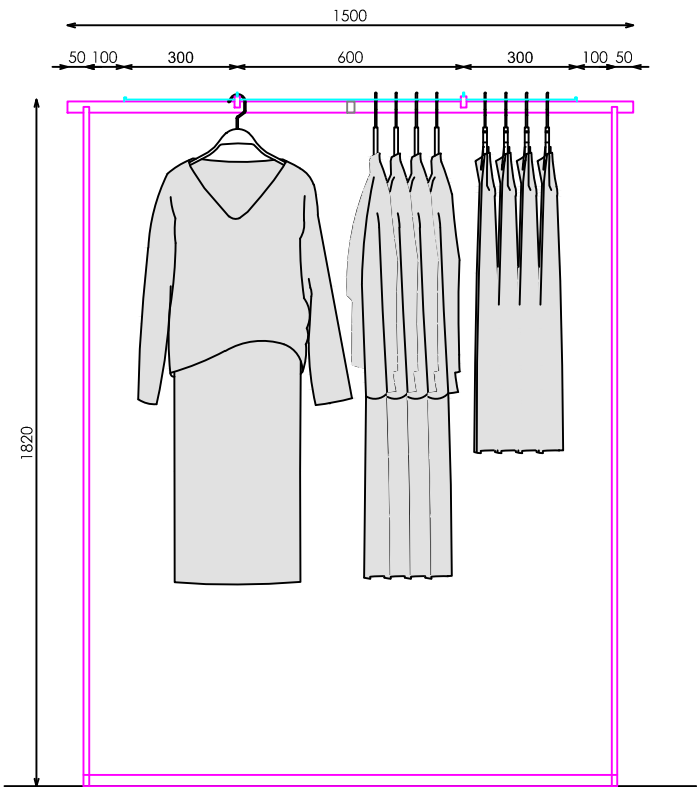
ALZADO
