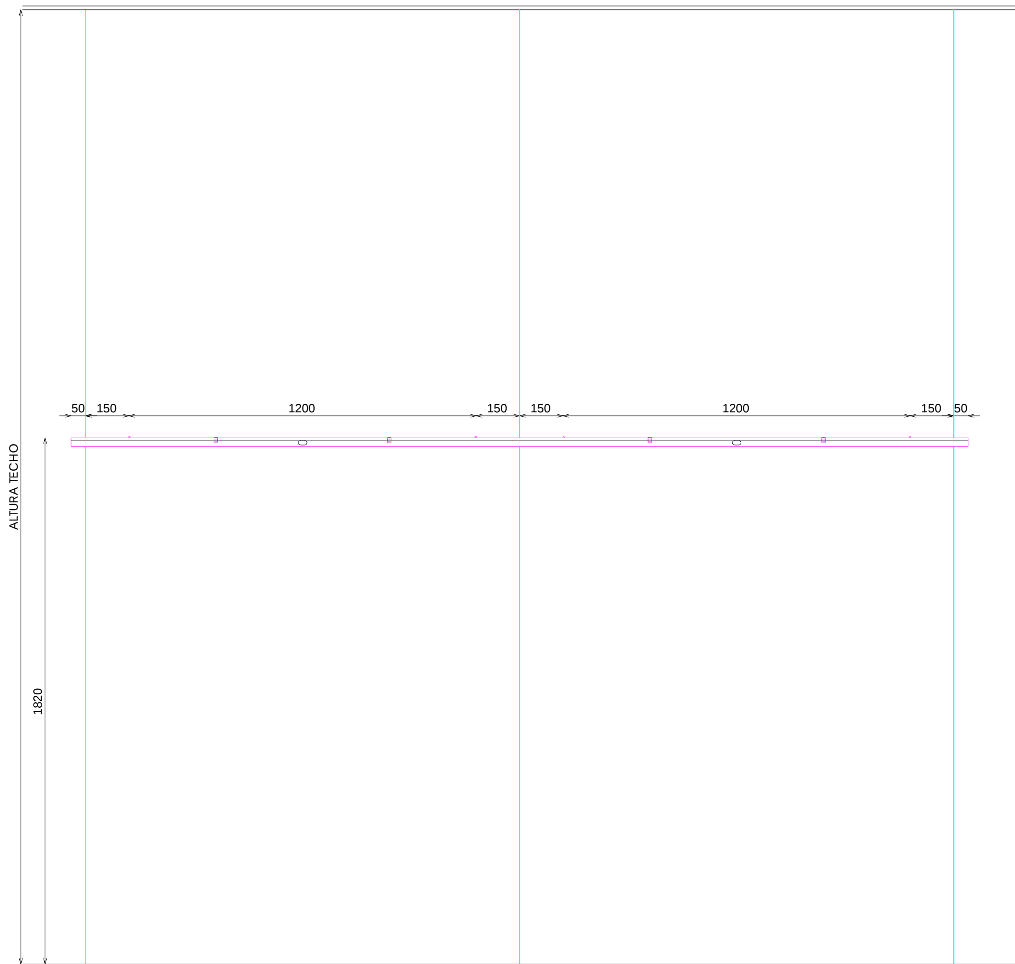
ALZADO FRONTAL
