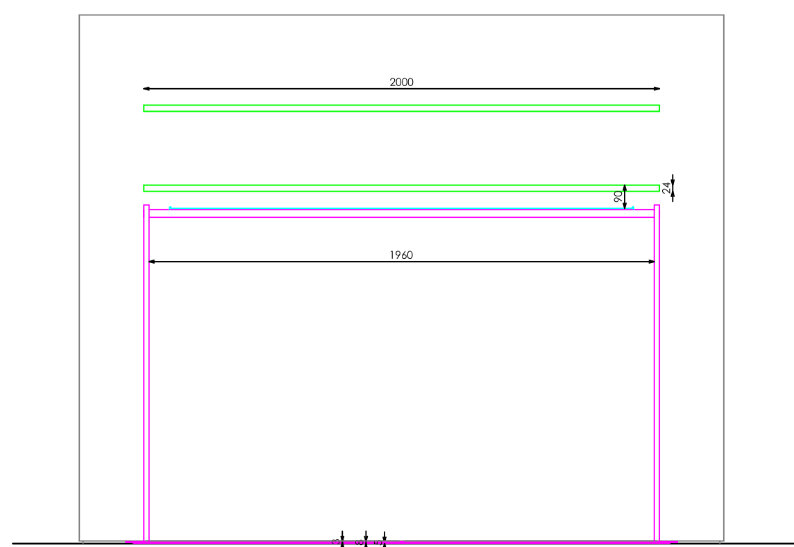
ALZADO
