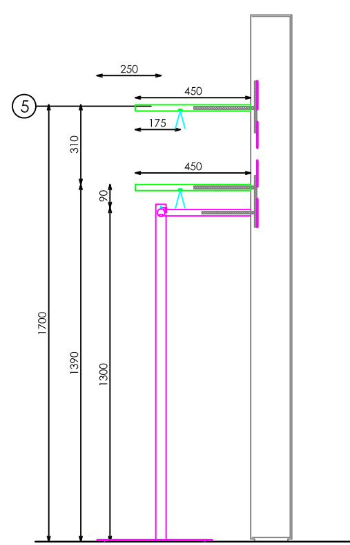
PERFIL
