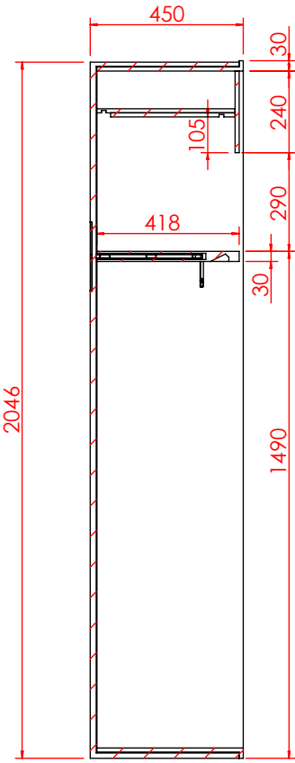
剖面 AJ-AJ
