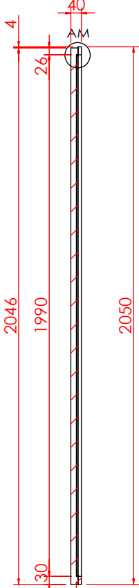
剖面 AL-AL
