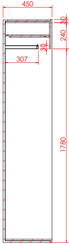
剖面 AK-AK
