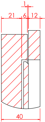
局部视图 AM 比例 1 : 2
