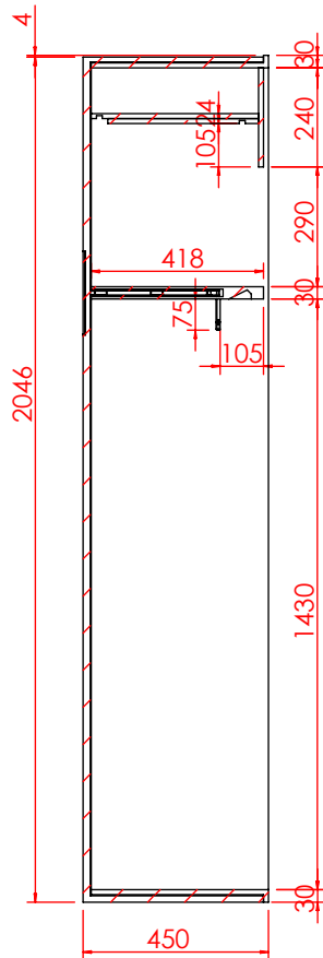
剖面 AG-AG
