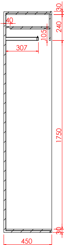
剖面 AH-AH
