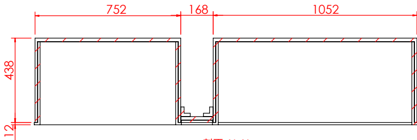
剖面 AI-AI
