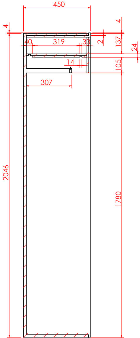
剖面 AG-AG
