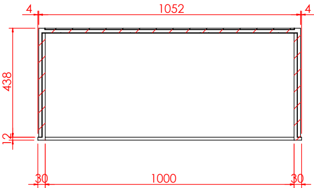
剖面 AJ-AJ
