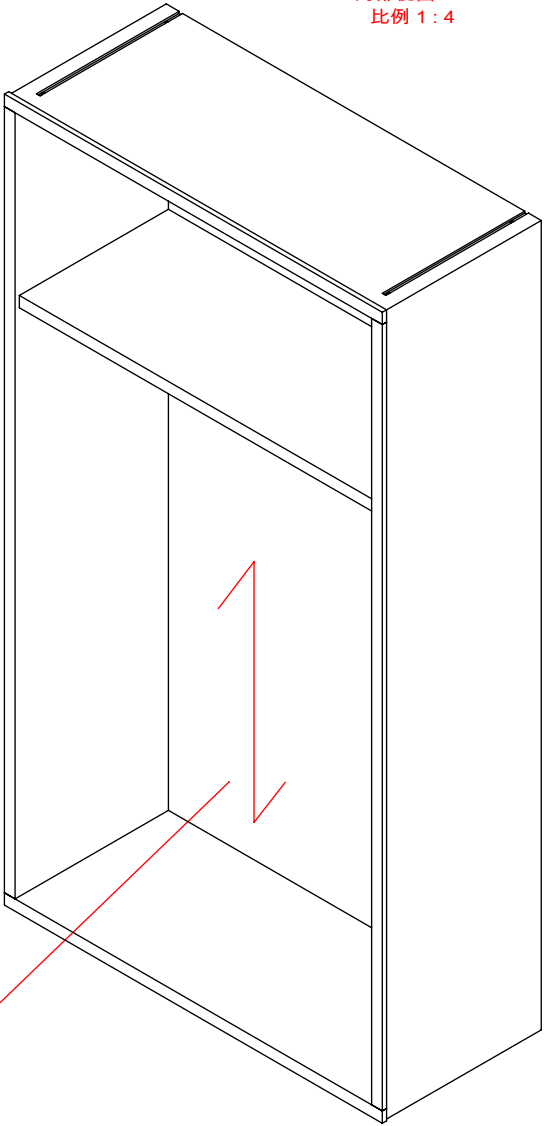
局部视图 AH 比例 1 : 4
