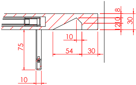
局部视图 AH 比例 1 : 4
