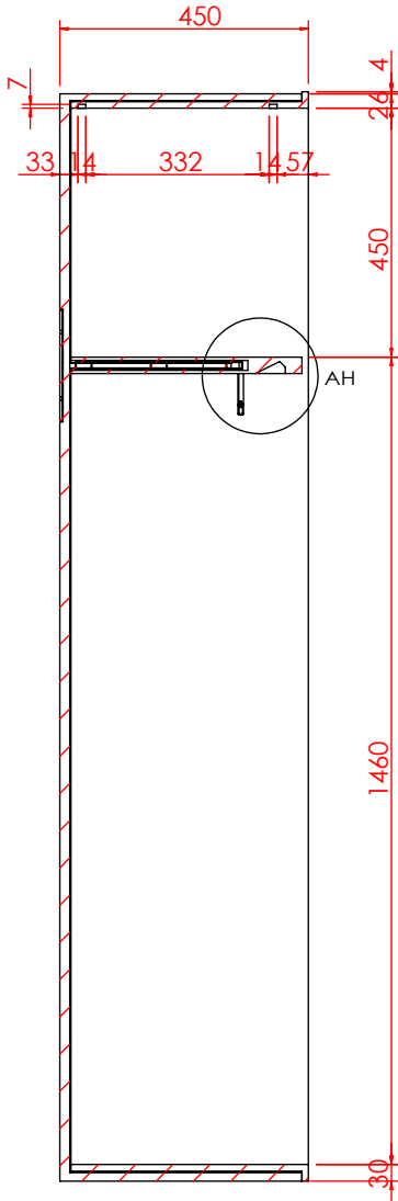
剖面 AG-AG
