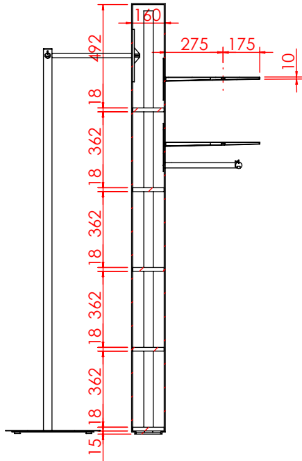
剖面 AG-AG
