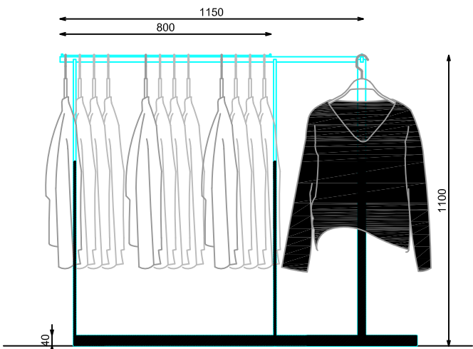
ALZADO FRONTAL
