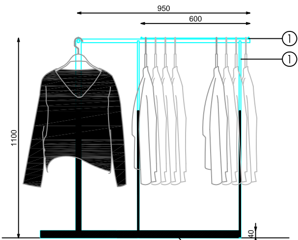
ALZADO LATERAL
