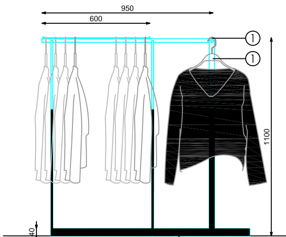
ALZADO LATERAL
