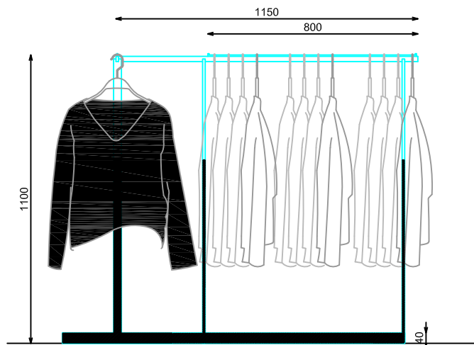
ALZADO FRONTAL
