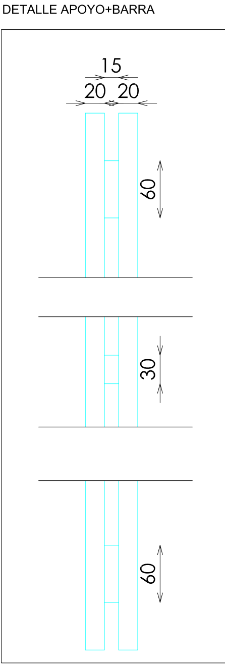
DETALLE APOYO+BARRA
