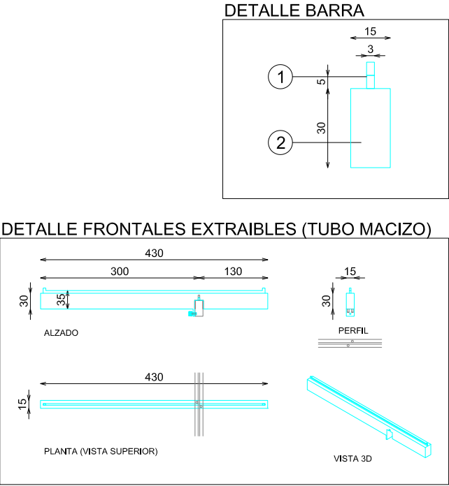
DETALLE BARRA
