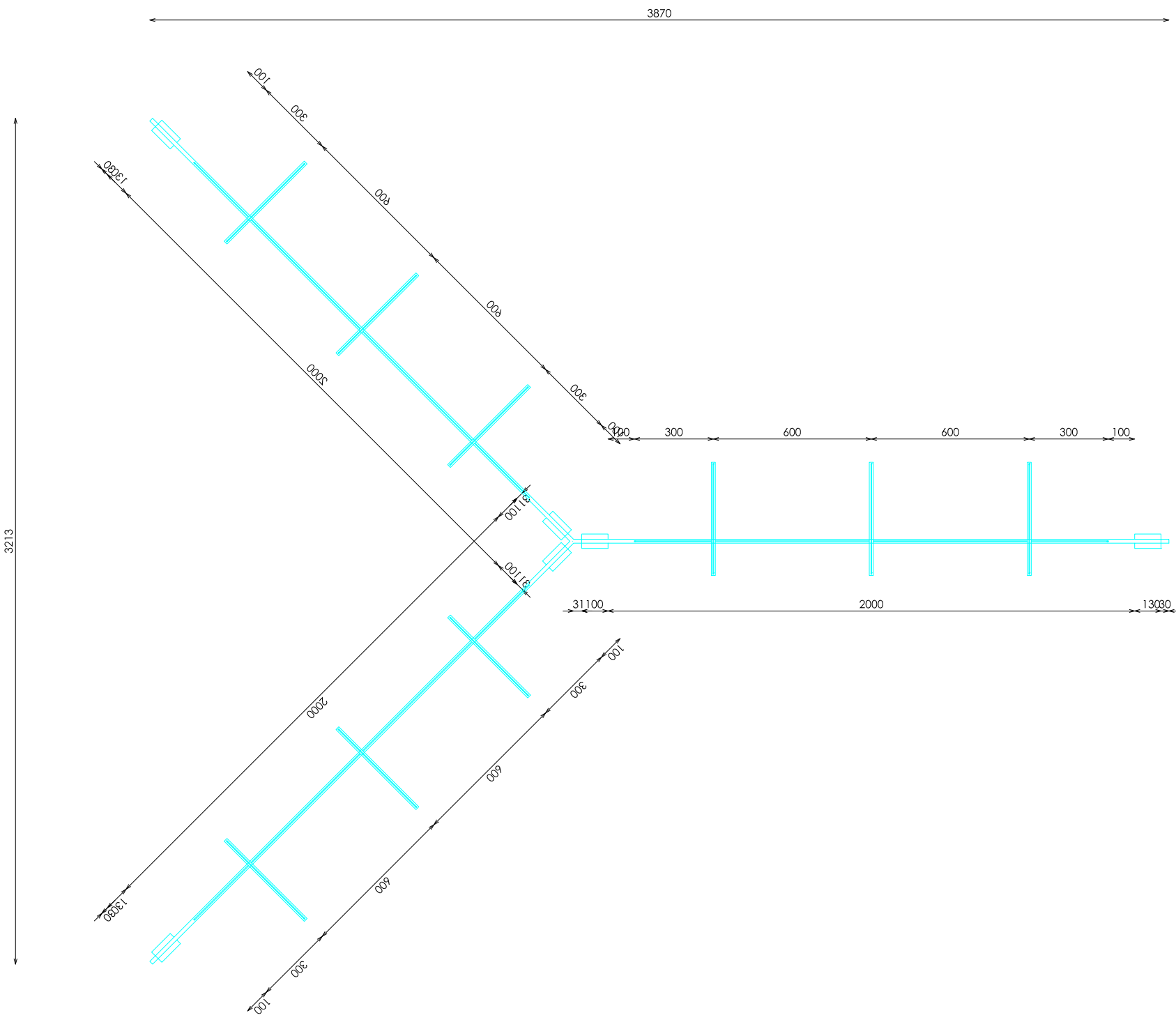
PLANTA
