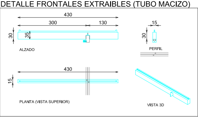
DETALLE FRONTALES EXTRAIBLES (TUBO MACIZO)
