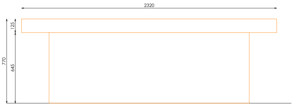
ALZADO
