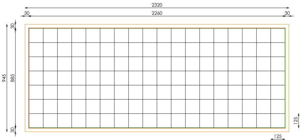
PLANTA
