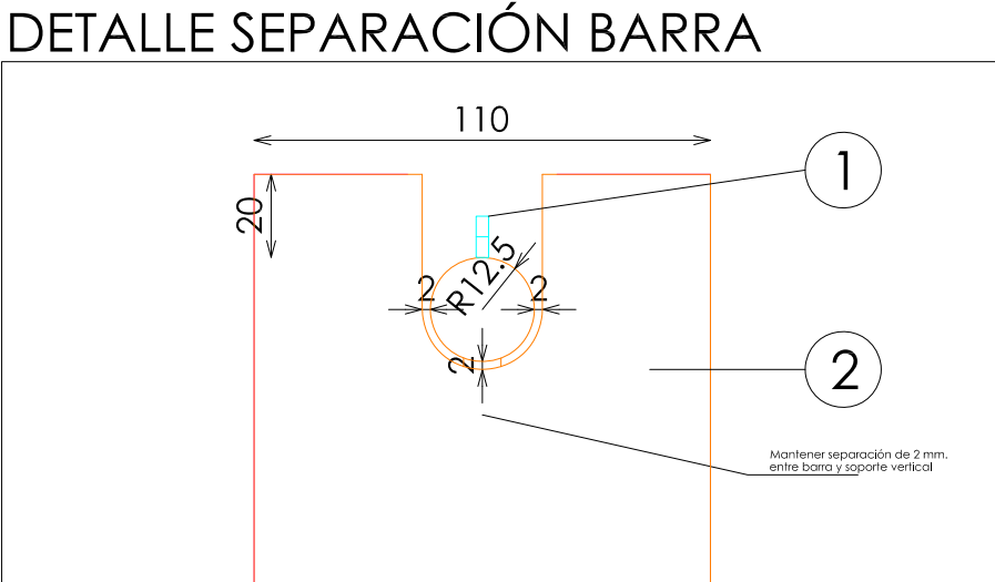
DETALLE SEPARACIÓN BARRA
