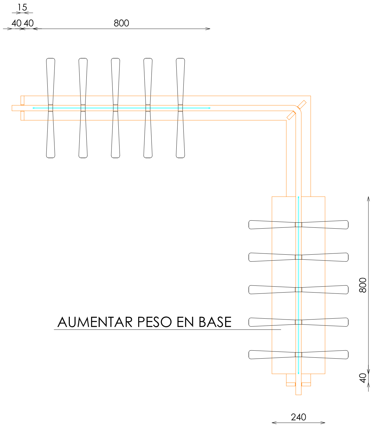
PLANTA
