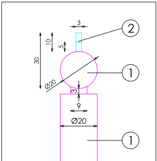
DETALLE ANTIROCE
