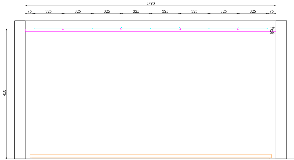
ALZADO FRONTAL
