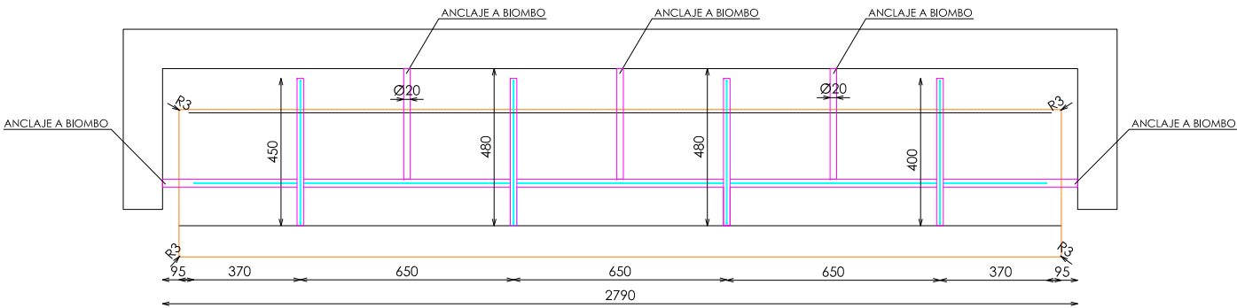
PLANTA
