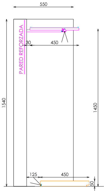
SECCIÓN
