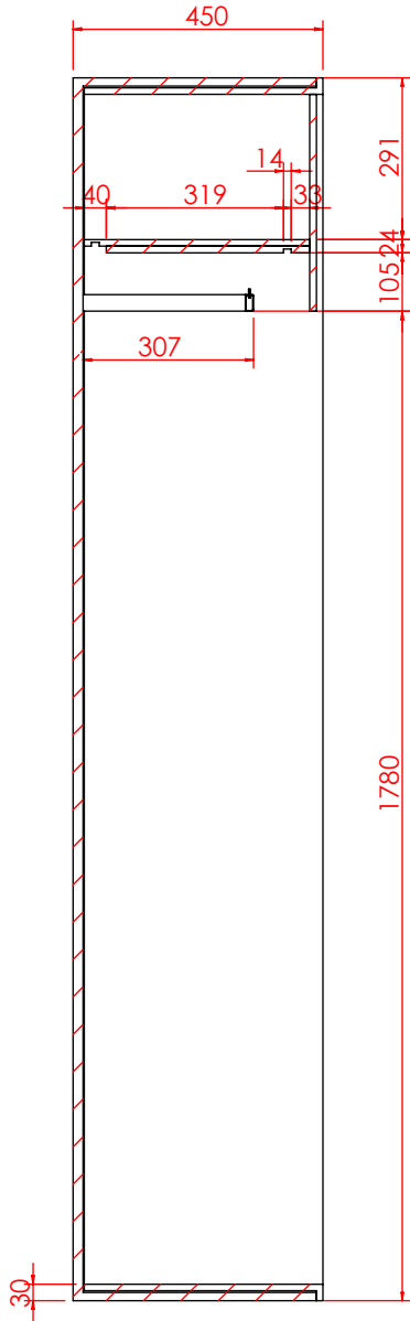
剖面 AG-AG
