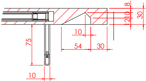
局部视图 AH 比例 1 : 4
