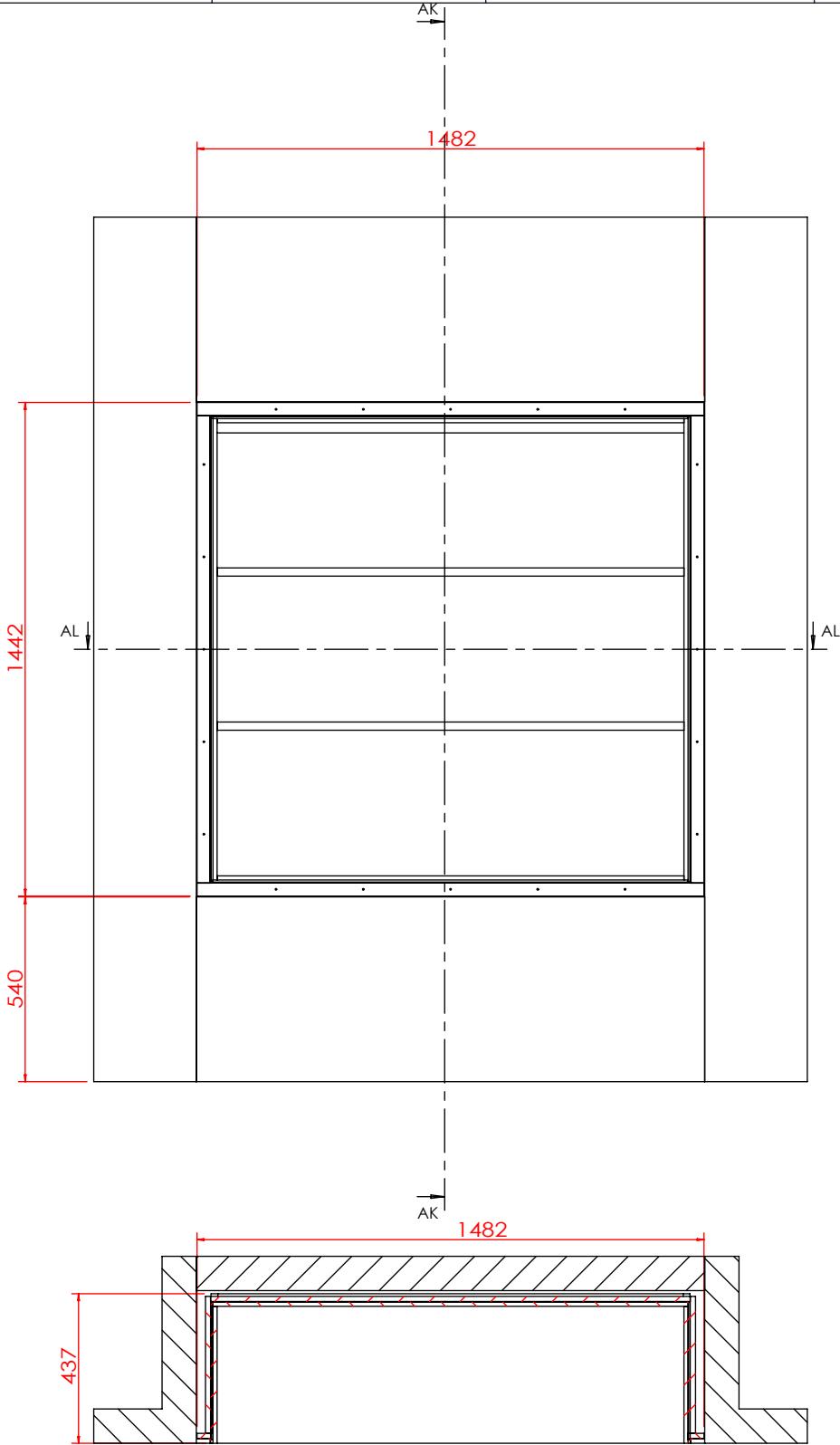
剖面 AL-AL
