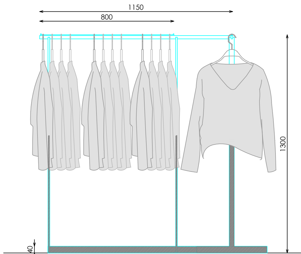
ALZADO FRONTAL
