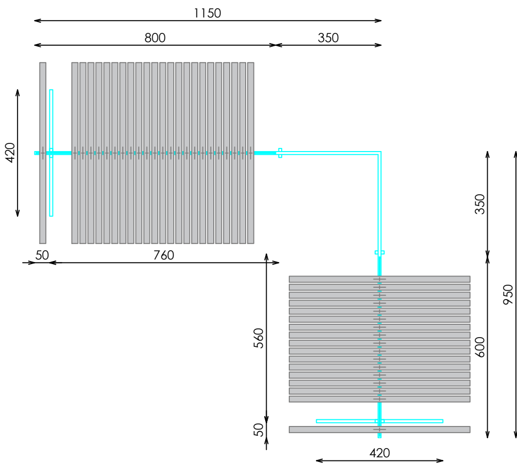
PLANTA
