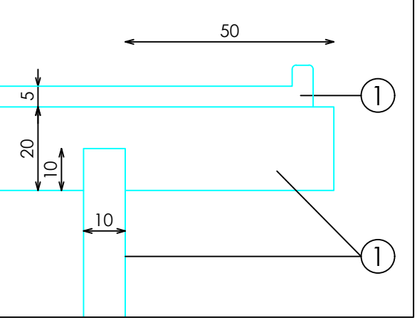
DETALLE C
