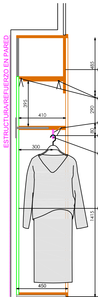
SECCIÓN BARRA H141 + ESTANTE
