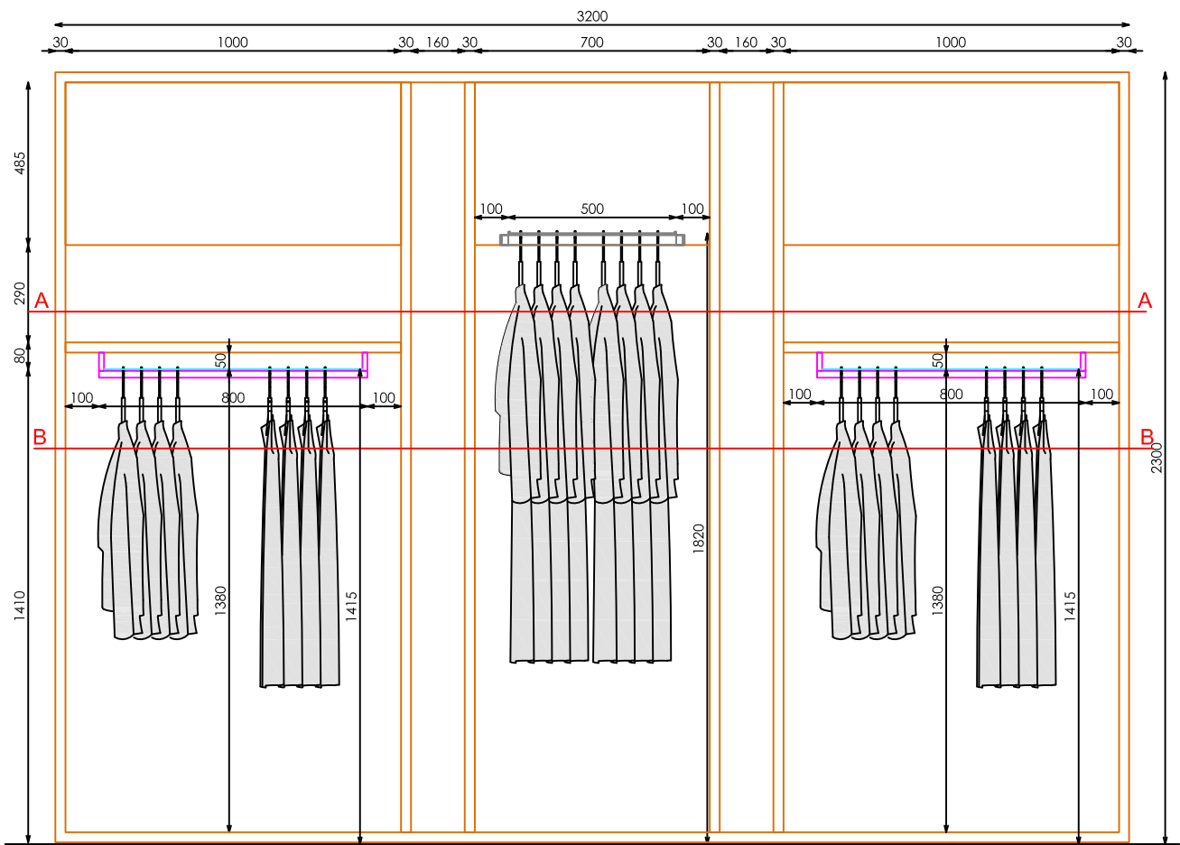
ALZADO
