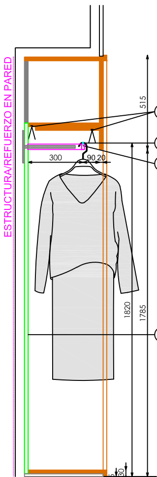
SECCIÓN BARRA H182
