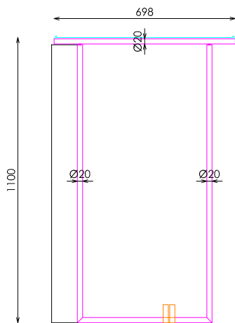
ALZADO
