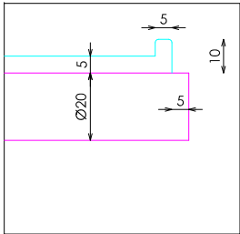
DETALLE B
