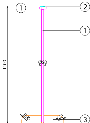
PERFIL
