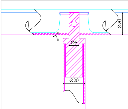
DETALLE C (SECCIÓN)
