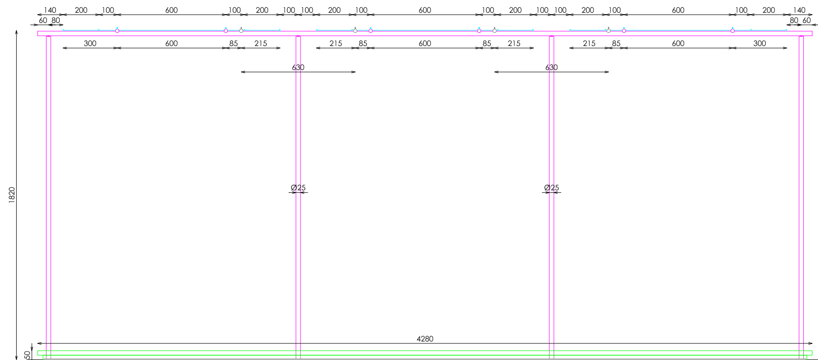
ALZADO FRONTAL
