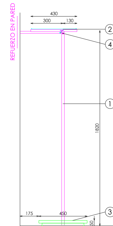
SECCIÓN
