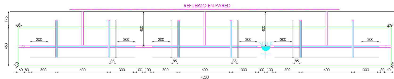
PLANTA
