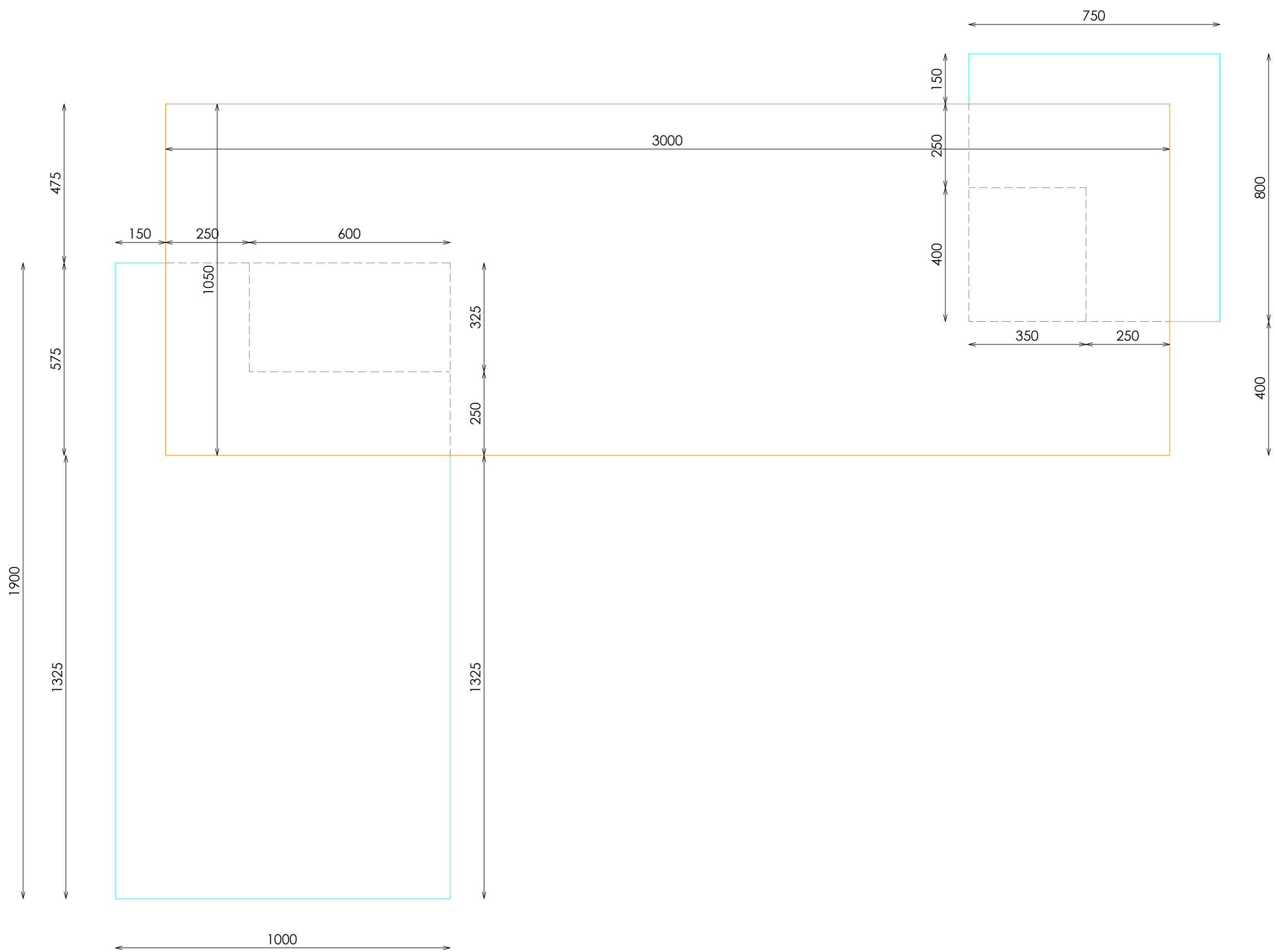
PLANTA
