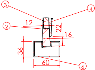
局部视图 AK 比例 1 : 5
