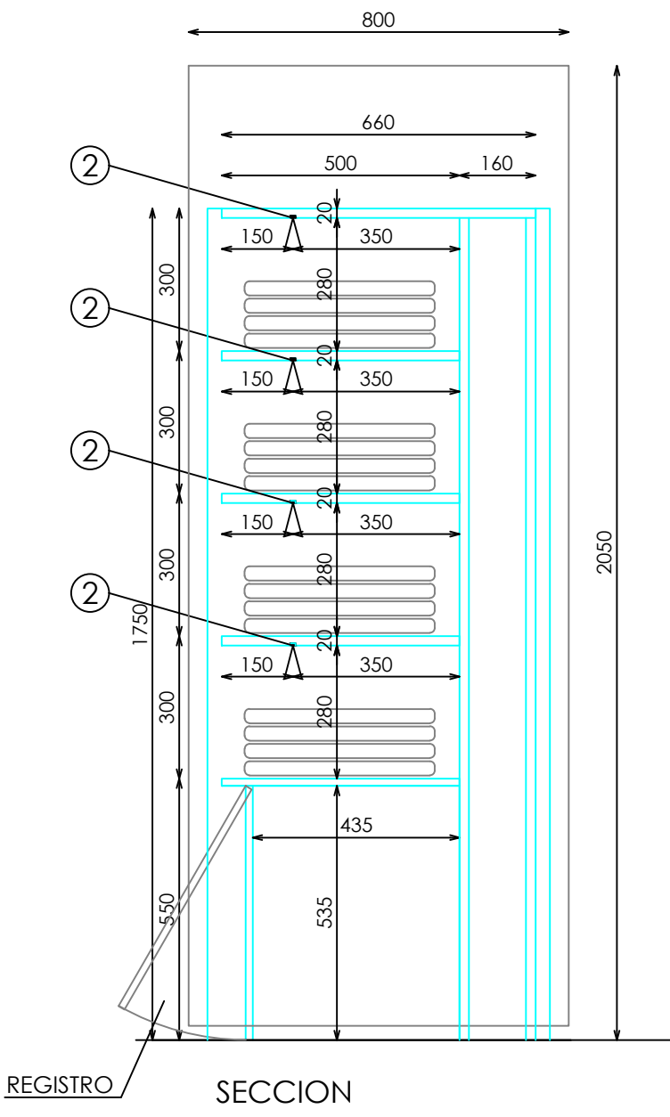
SECCION
