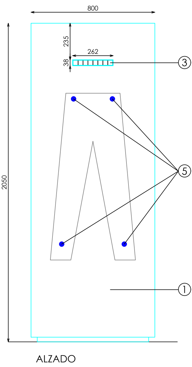
ALZADO
