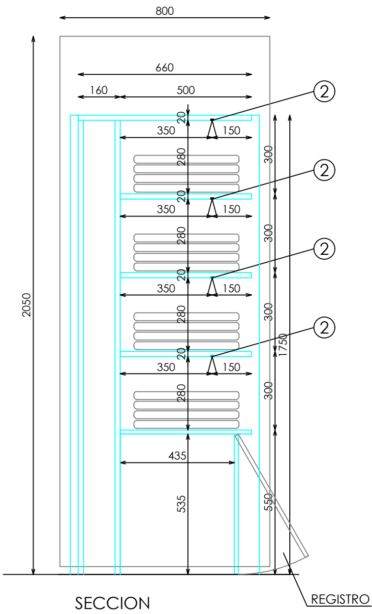
SECCION
