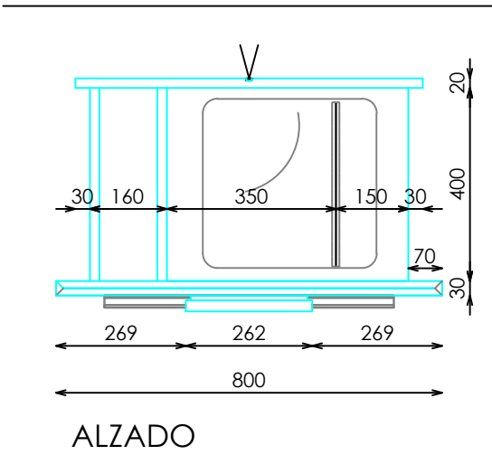
ALZADO
