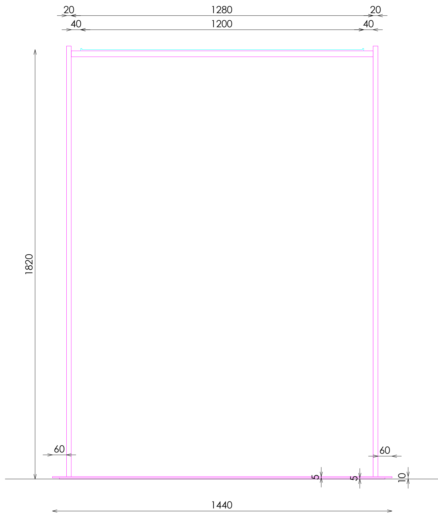
ALZADO
