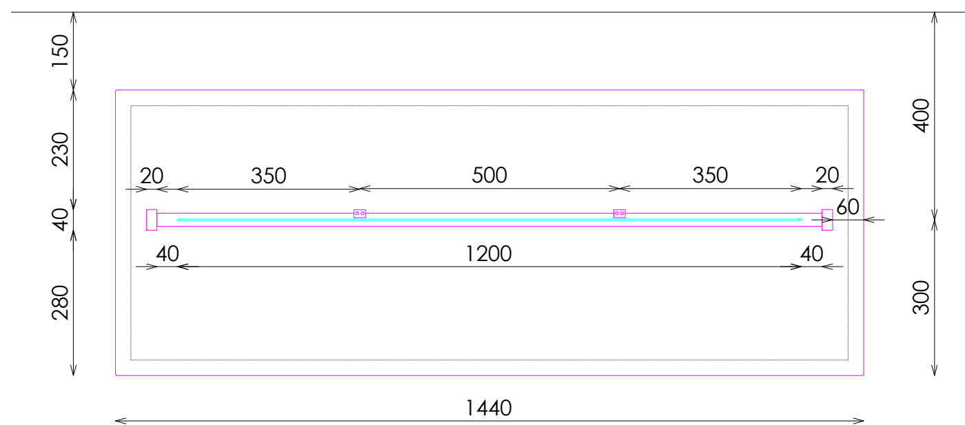
PLANTA
