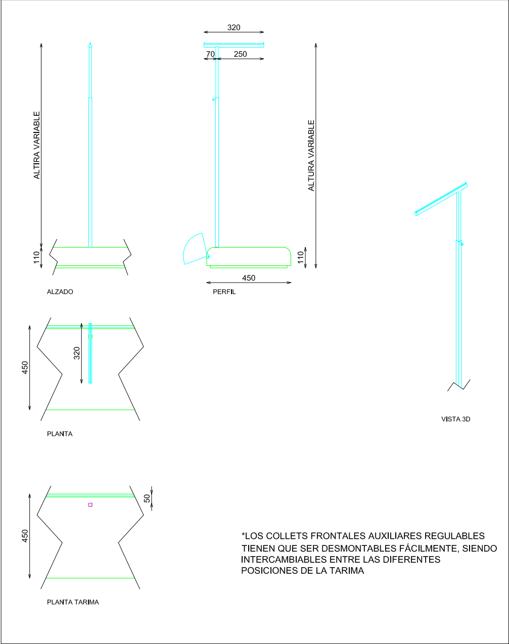
DOTACION COLGADOR AUXILIAR REGULABLE (2 UDS)
