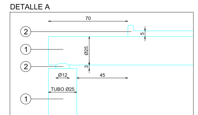
DETALLE ILUMINACION TARIMA
