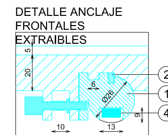
DETALLE A
