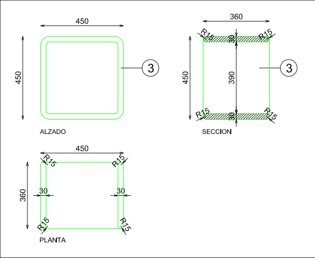
DOTACION BANCO 45x36xH45 (2 UDS)
