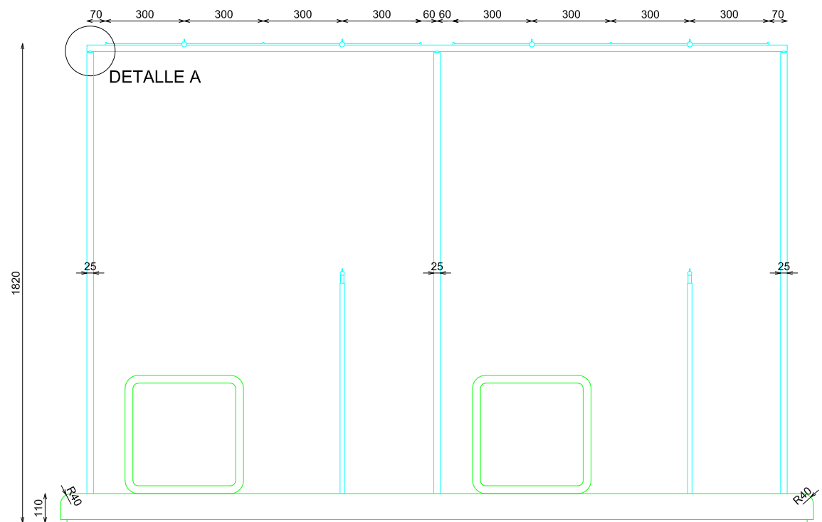
ALZADO FRONTAL
