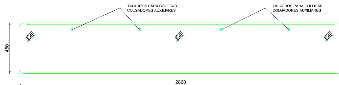
PLANTA SECCIONADA (ILUMINACIÓN EN TARIMA)
