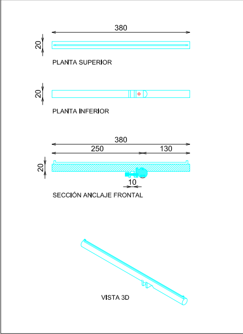
FRONTAL EXTRAIBLE. TUBO MACIZO (4 UDS)
