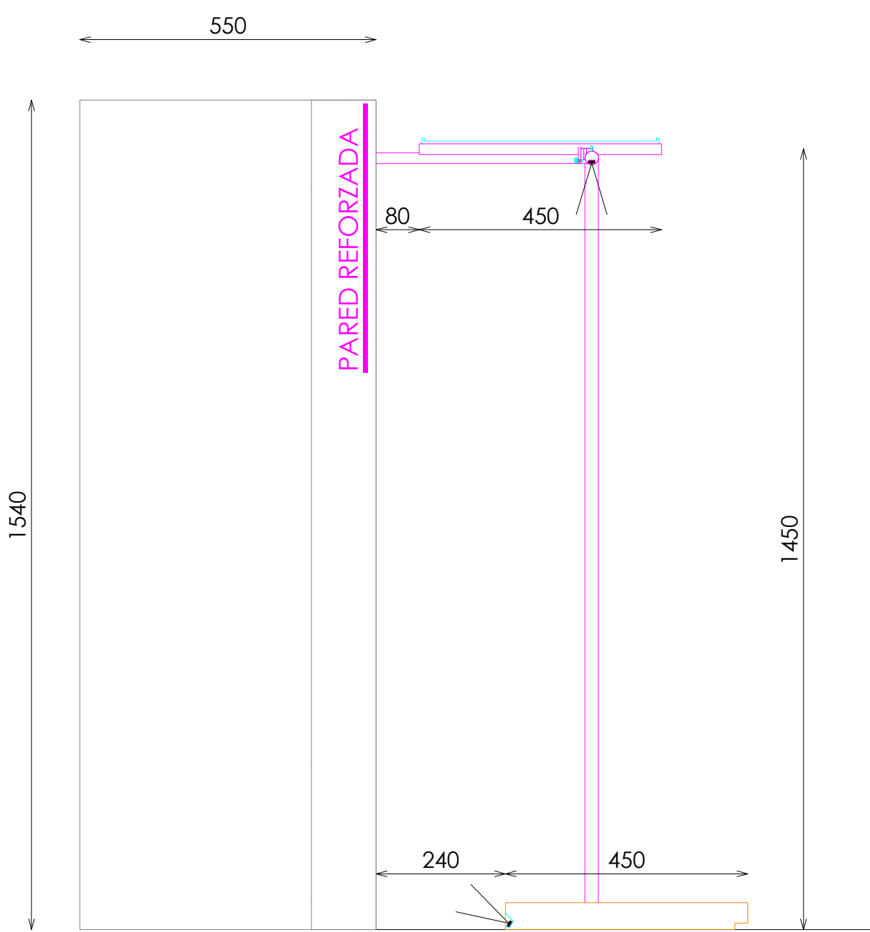
SECCIÓN
