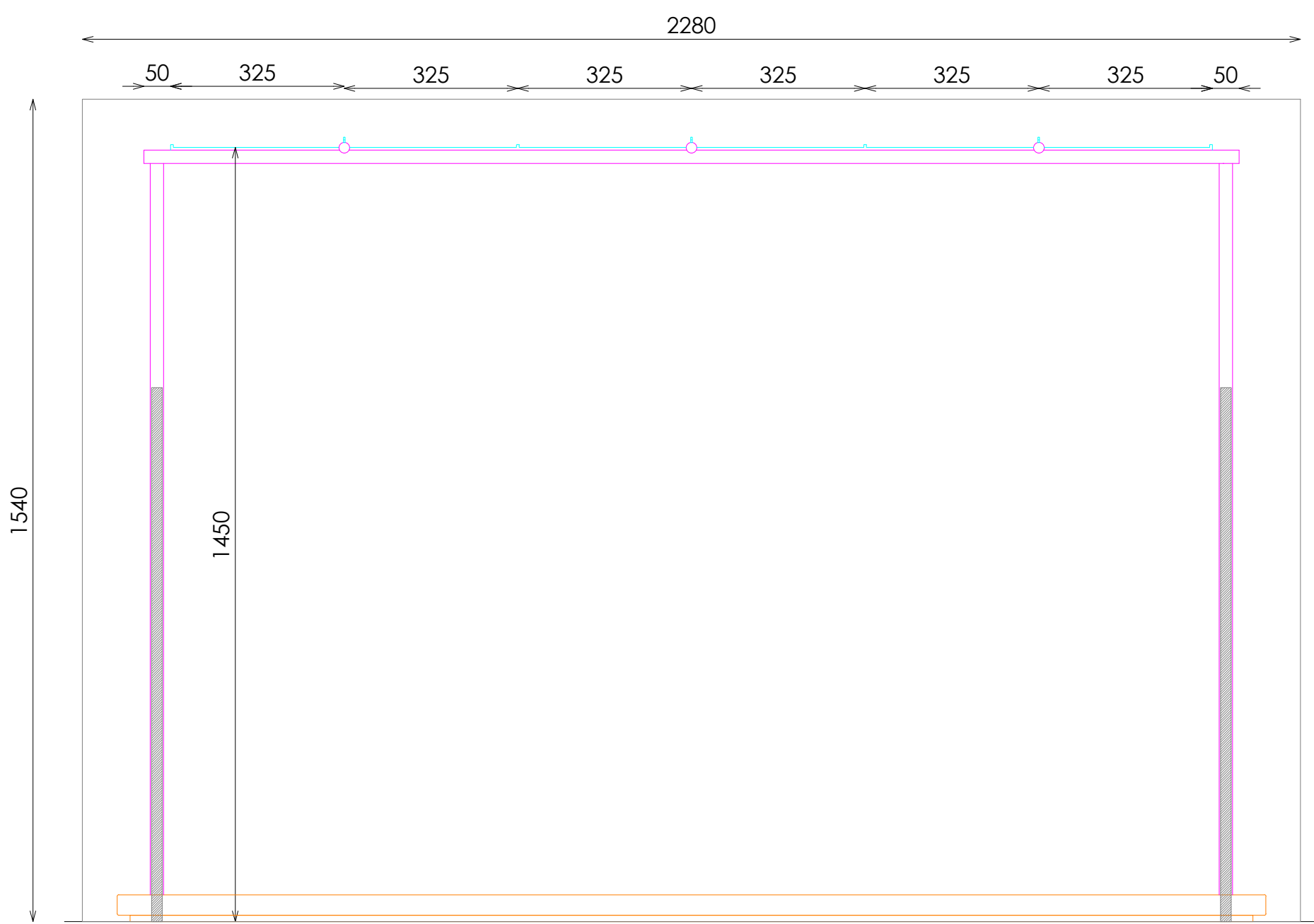
ALZADO FRONTAL
