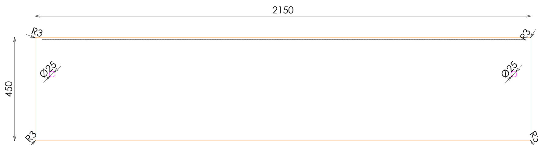
PLANTA TARIMA
