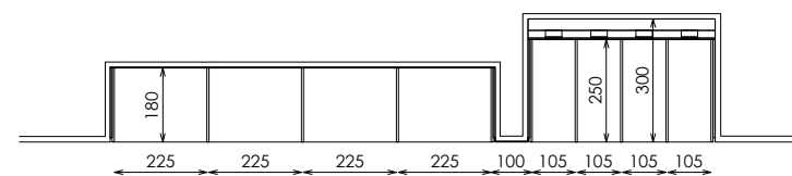
PLANTA A-A
