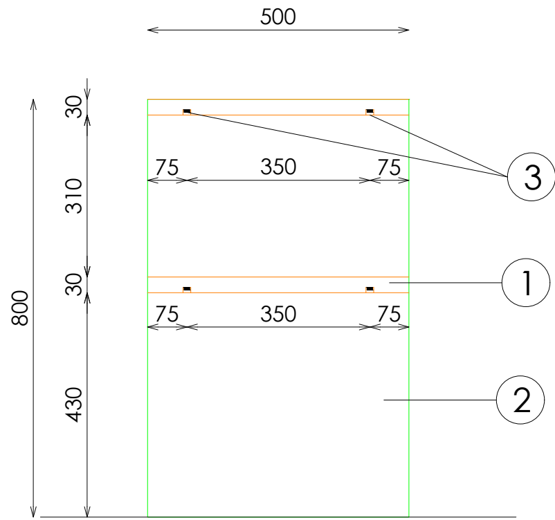
SECCIÓN
