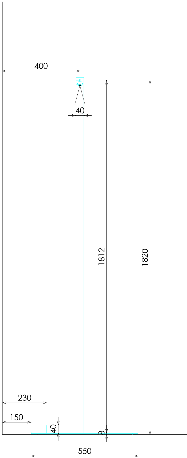
PERFIL SECCIONADO
