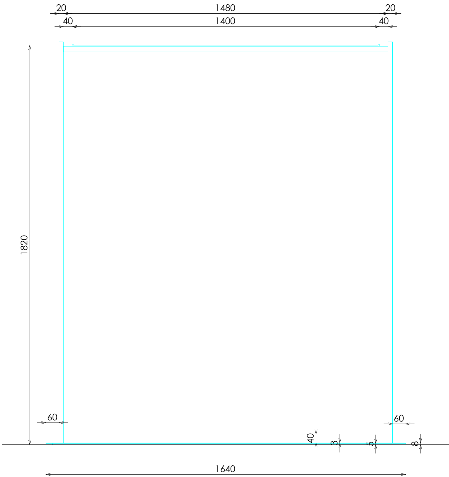
ALZADO SECCIONADO
