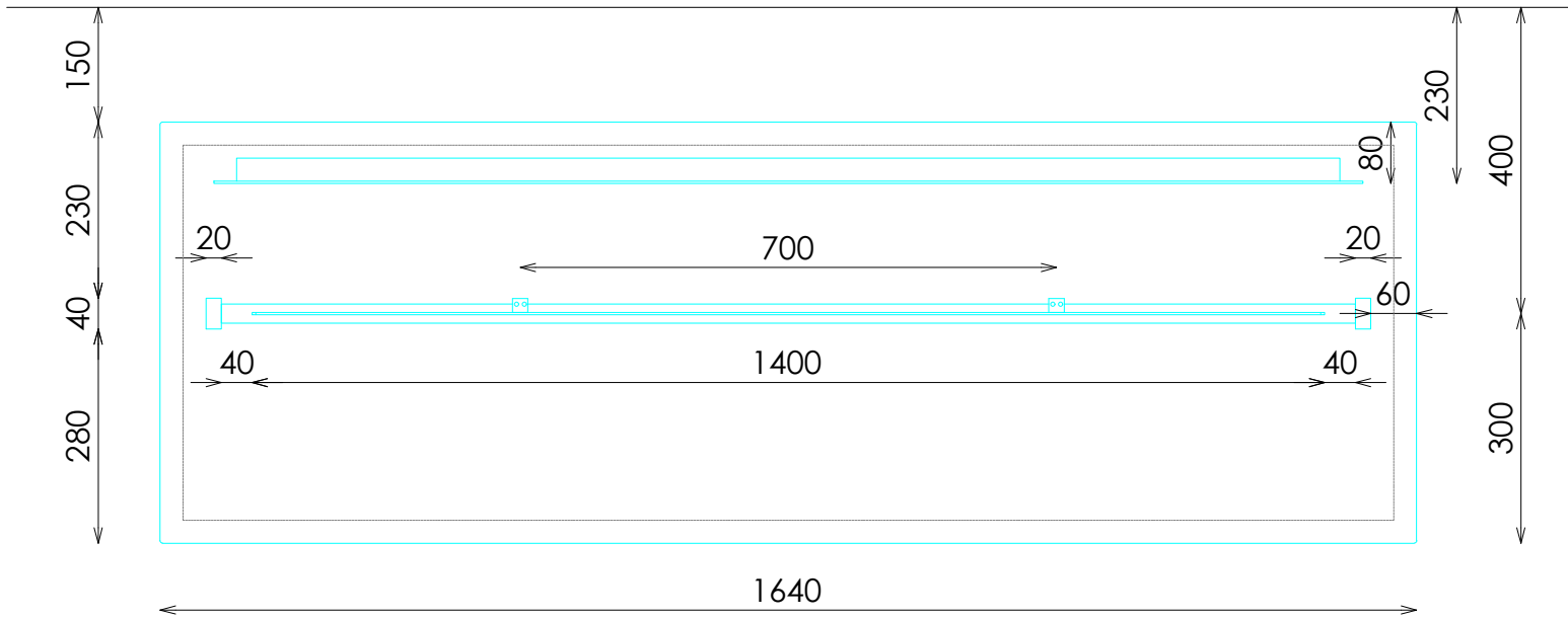
PLANTA
